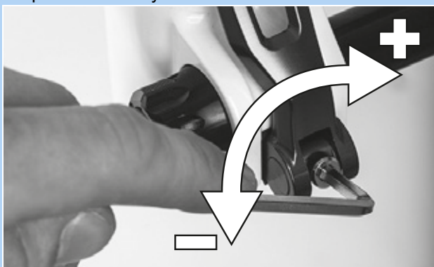
Rysunek 110: Ustawianie siły mocowania zacisku szybko mocującego
