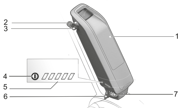
Rysunek 23: Szczegóły akumulatora zintegrowanego z ramą
