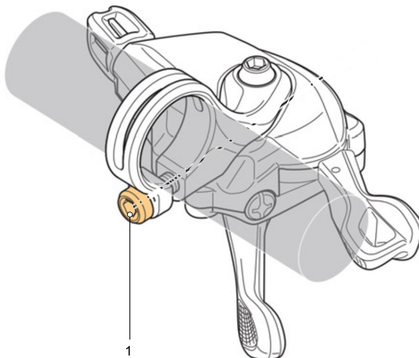
Rysunek 68: Położenie śruby mocującej dźwignię przerzutki SHIMANO
