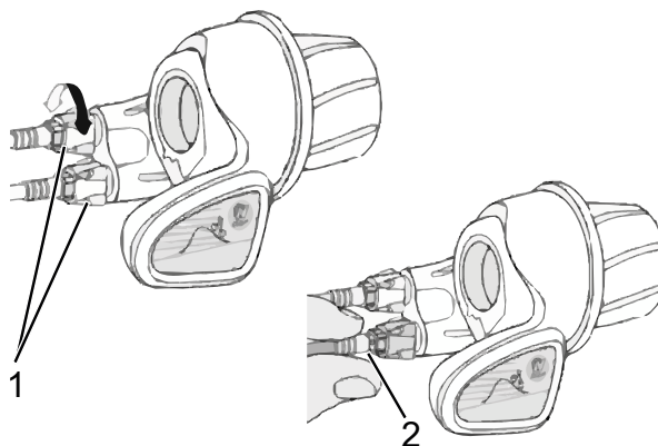
Rysunek 108: Manetka obrotowa z nakrętkami regulacyjnymi (1) i luzem mechanizmu zmiany przerzutek (2)
