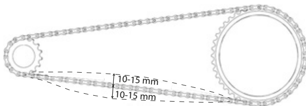
Rysunek 103: Kontrola naprężenia łańcucha
