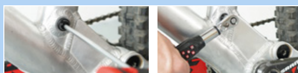
Rysunek 142: Mocowanie osi sworznia
