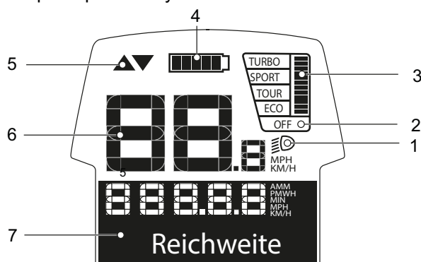
Rysunek 32: Zestawienie wskaźników komputera pokładowego
