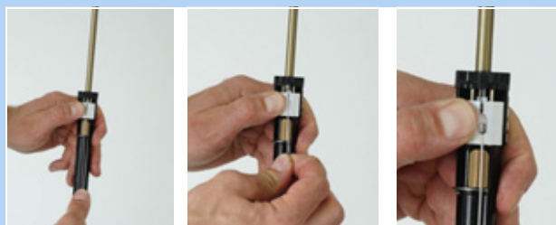
Rysunek 117: Odczepianie linki
