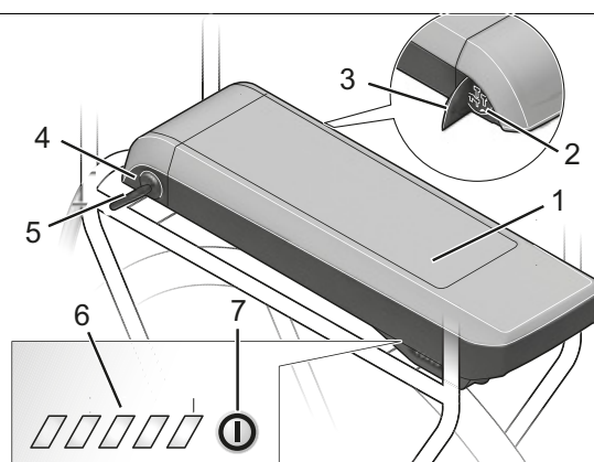
Rysunek 25: Szczegóły akumulatora zintegrowanego z bagażnikiem
