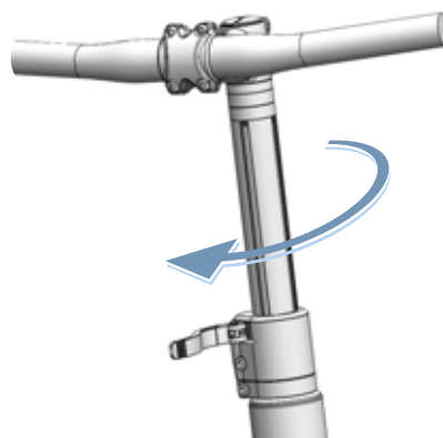
Rysunek 94: Przykład skręconej kierownicy typu All Up
