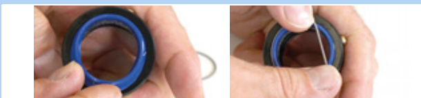
Rysunek 161: Wkładanie i mocowanie zgarniacza
