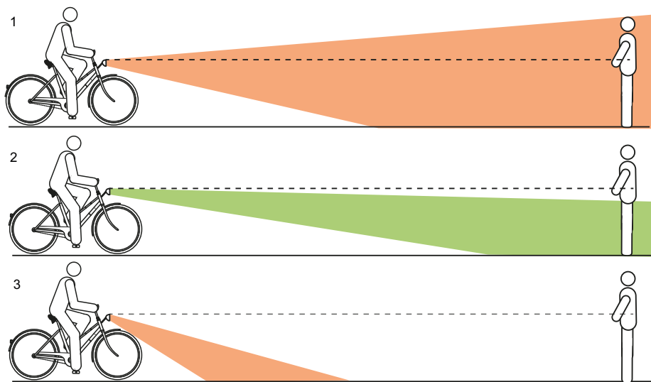
Rysunek 69: Światło ustawione za wysoko (1), prawidłowo (2) i za nisko (3)
