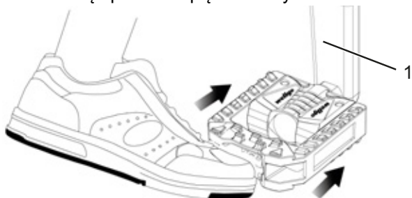
Rysunek 84: Dociskanie pedału do korby (1)
