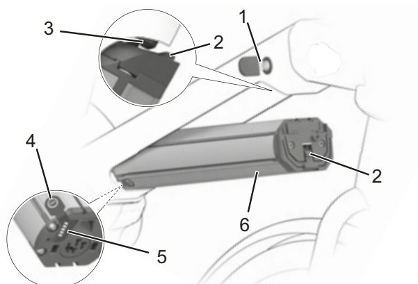
Rysunek 27: Szczegóły zintegrowanego akumulatora
