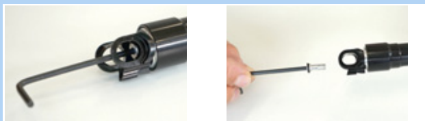
Rysunek 132: Odkręcanie nakrętki zaworu
