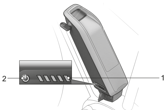
Rysunek 36: Pozycja wskaźnika stanu naładowania na akumulatorze na ruszce podsiodłowej
