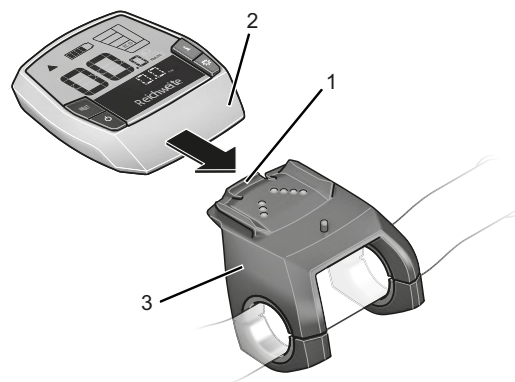
Rysunek 72: Wsunąć komputer pokładowy (2) przez blokadę (1) tego urządzenia do oporu w uchwyt (3)
